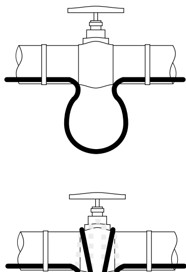
Прокладка вдоль вентилях
