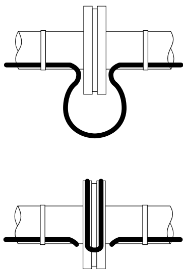
Прокладка вдоль фланцев
