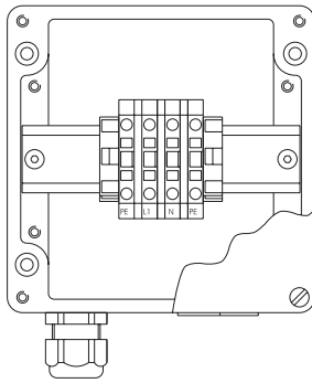
Anschlussgehäuse Ex 300
