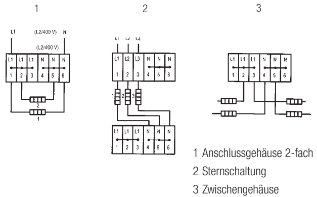
Schaltbild für Anschlussgehäuse Ex 400 S
