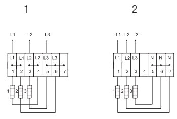
Schaltbild für Anschlussgehäuse Ex 690 S/D
