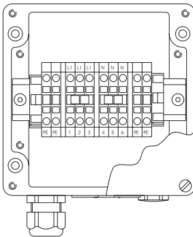
Anschluss-/Abschlussgehäuse Ex 400 S
