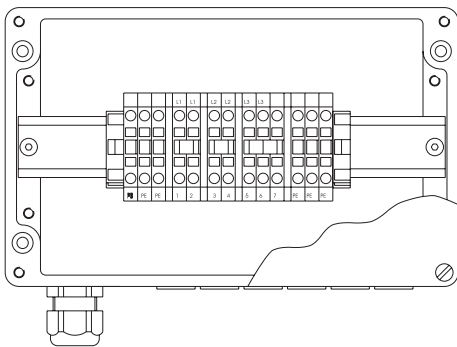
Anschlussgehäuse Ex 400 D
