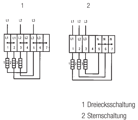
Schaltbild für Anschlussgehäuse Ex 400 D
